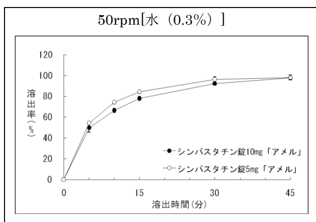
図. 溶出曲線
