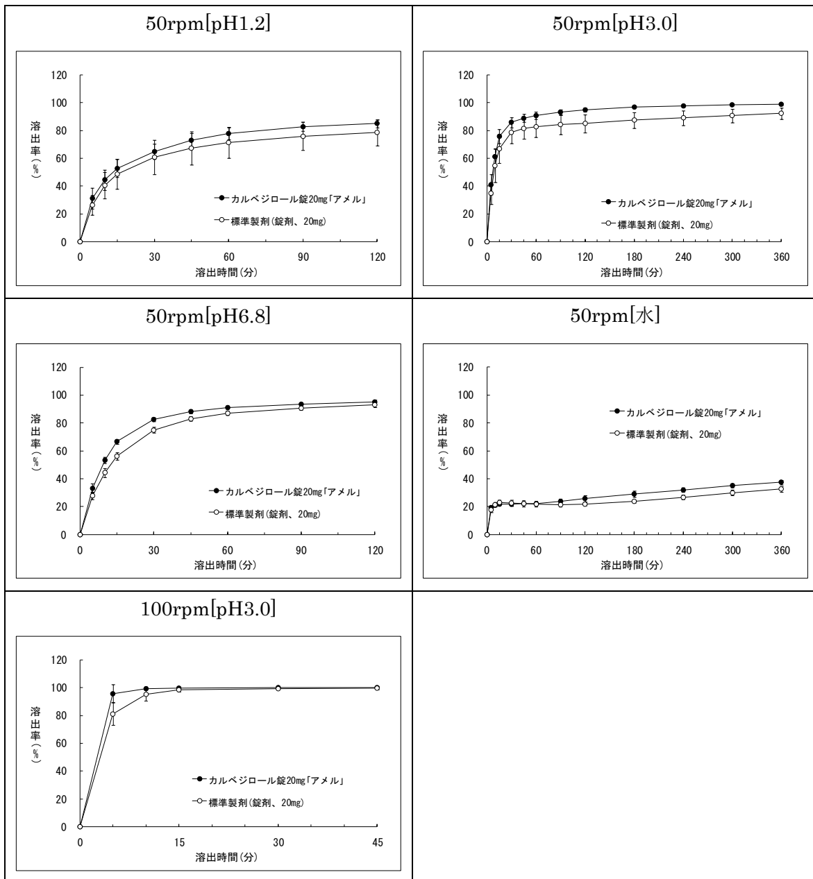
図 1. 溶出曲線
