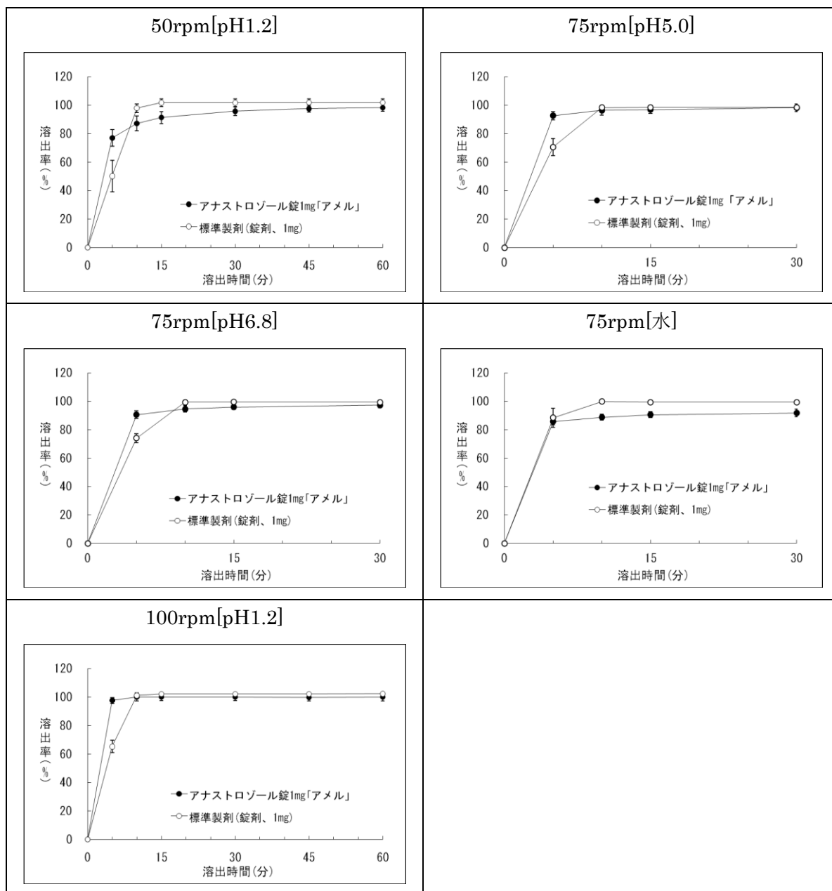
図 1. 溶出曲線
