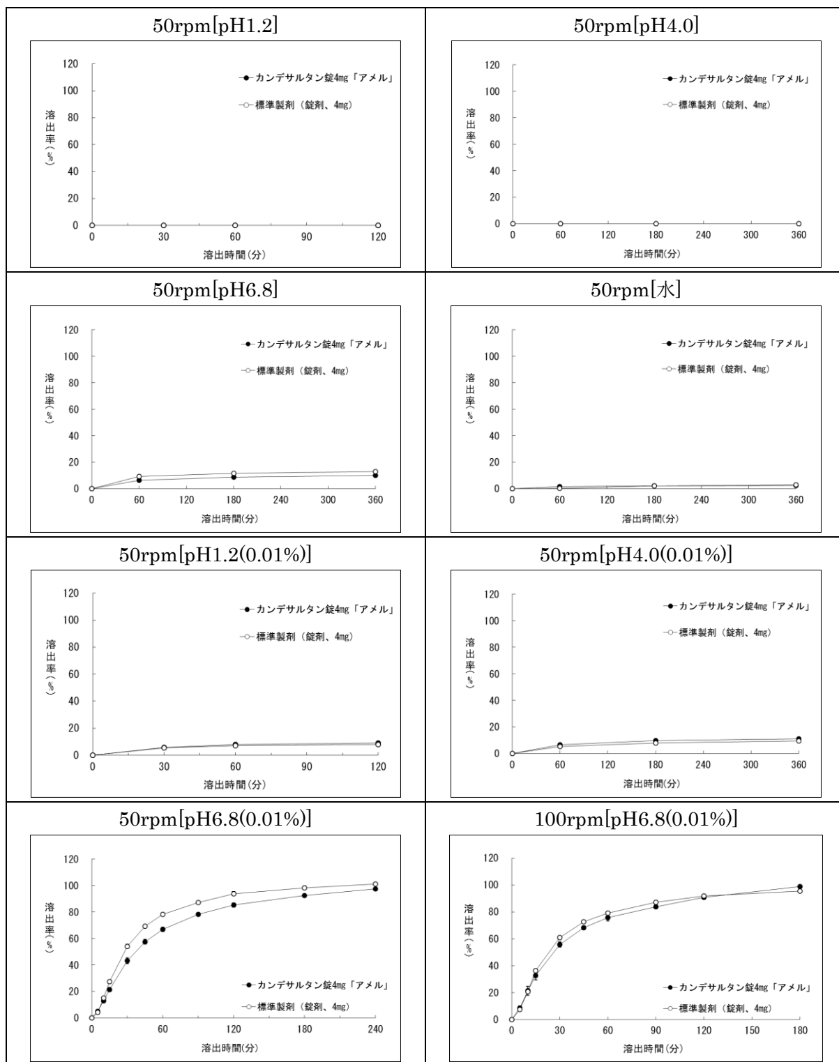
図 1. 溶出曲線
