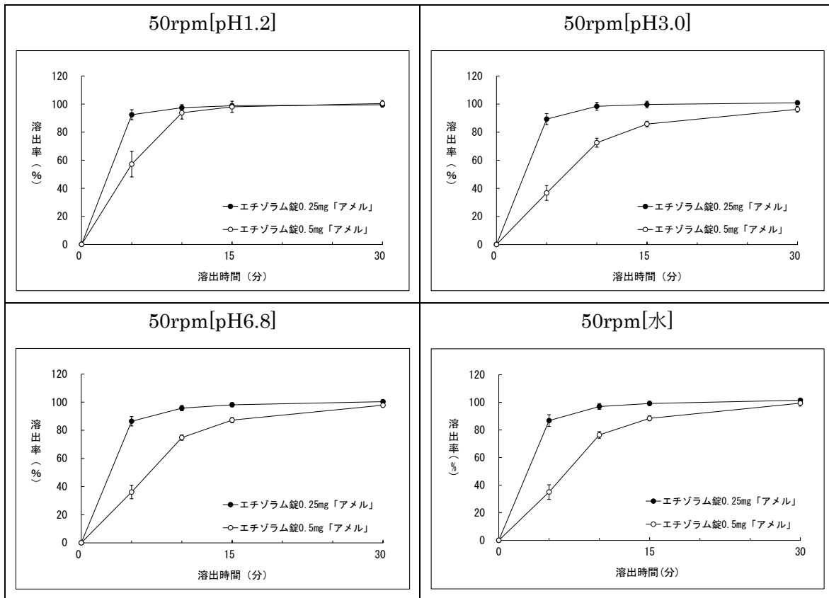
図 1. 溶出曲線
