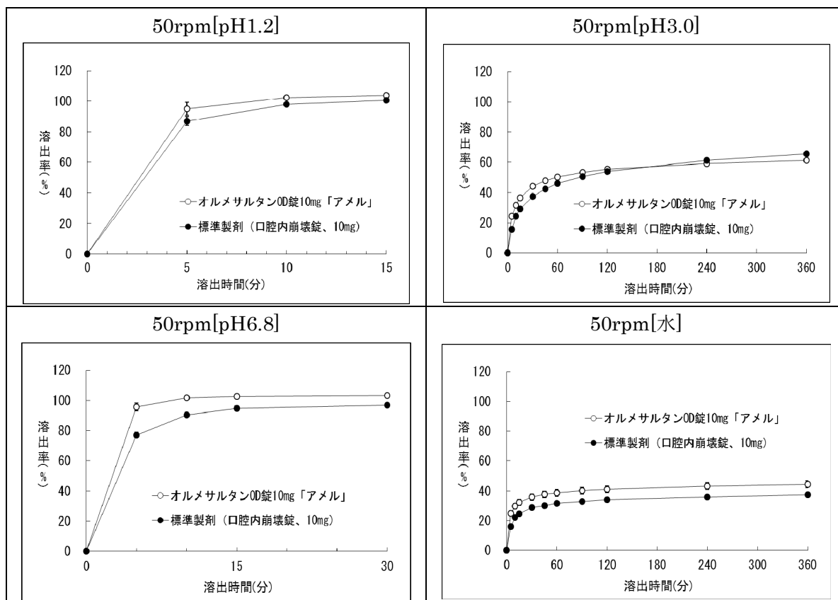
図 2. 溶出曲線
